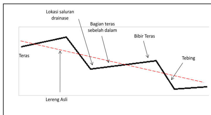
Gambar 9. Sketsa Guludan pada Lahan Berlereng < 8\%
